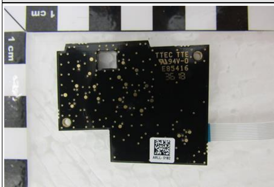
R-Sensor PCB Bottom
