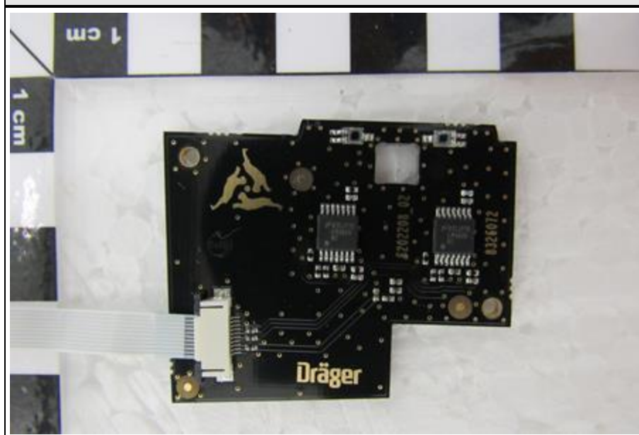
R-Sensor PCB Top
