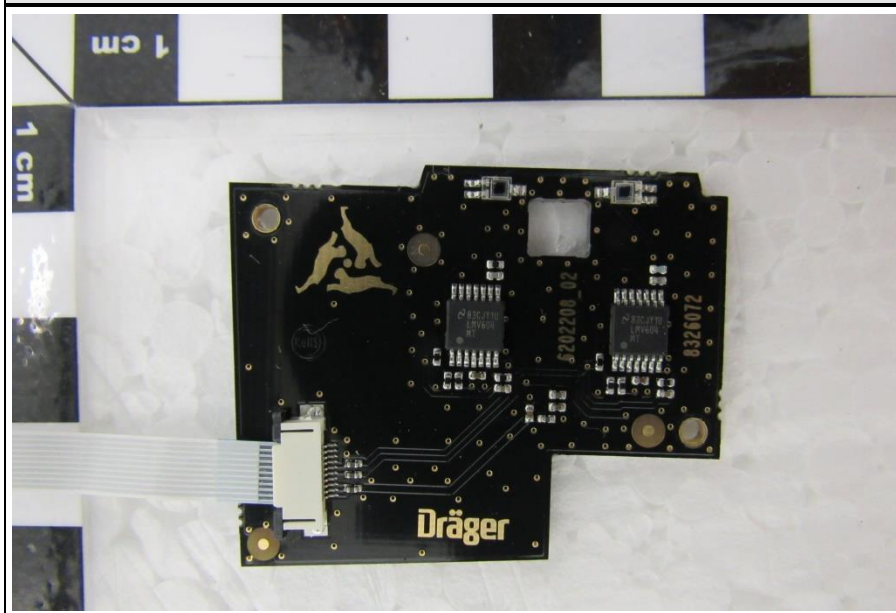
R-Sensor PCB Top
