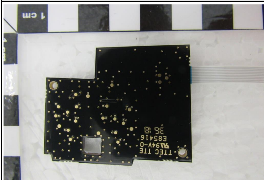
L-Sensor PCB Bottom
