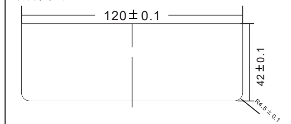
结构图纸
