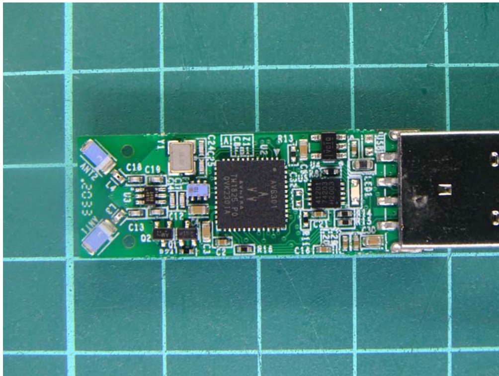
(13) EUT Photo
