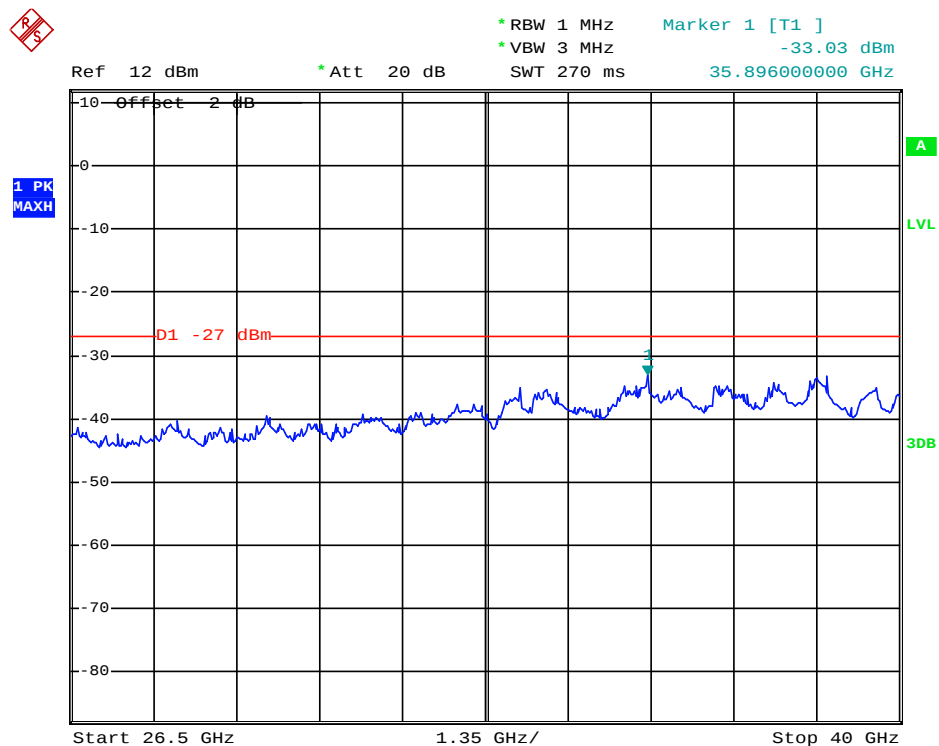
(Plot 4.9.1 B7: Channel 40: 5200MHz @ 802.11a)
