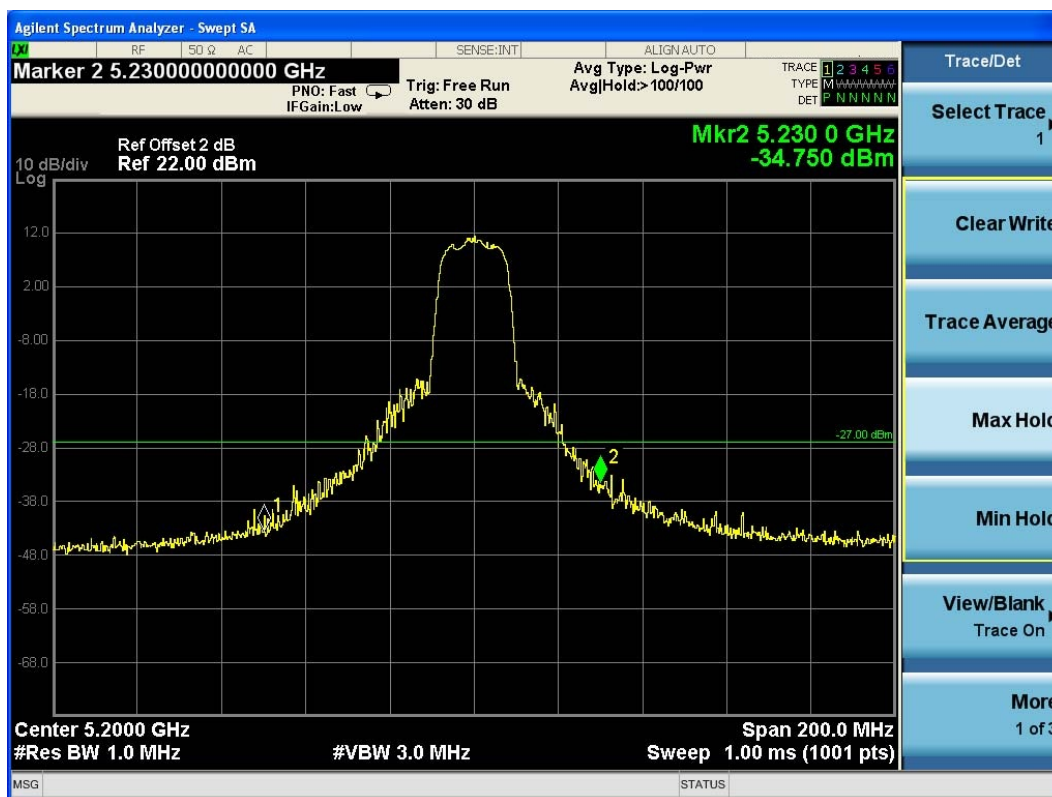
(Plot 4.9.1 B1: Channel 40: 5200MHz @ 802.11a)
