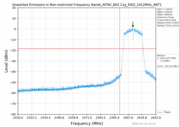
802.11g_2412MHz_SISO_ANT1
