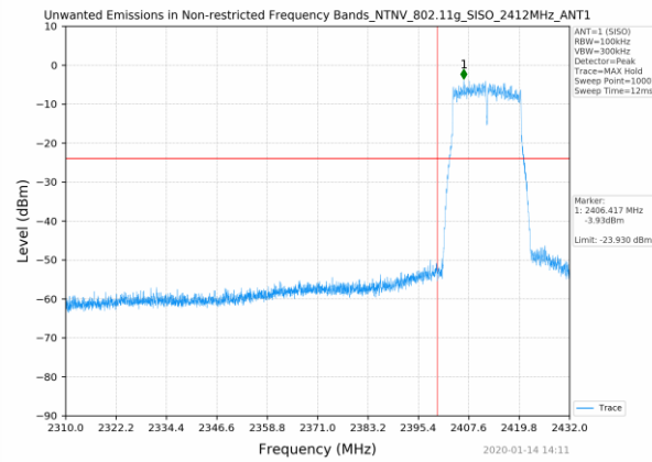
802.11g_2412MHz_SISO_ANT1
