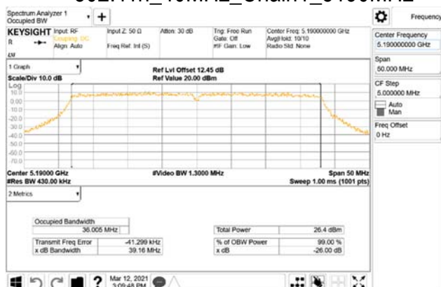
802.11n_40MHz_Chain1_5190MHz
