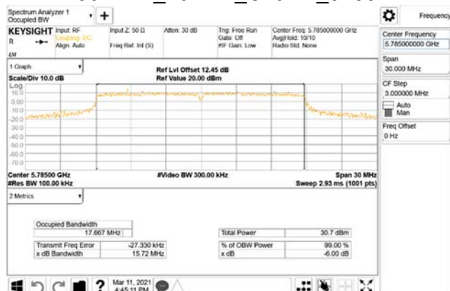
802.11n_20MHz_Chain1_5785MHz
