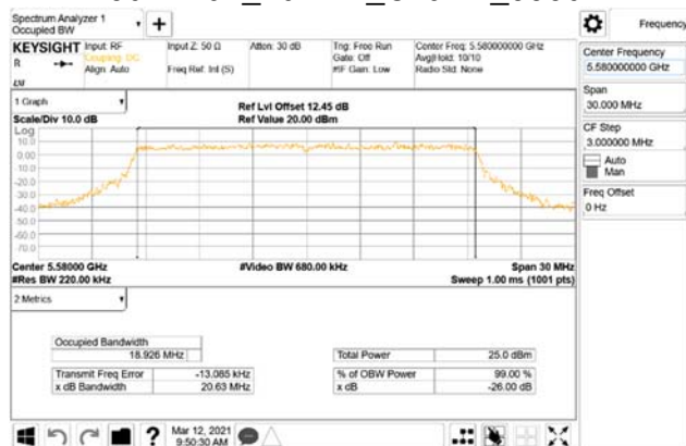
802.11ax_20MHz_Chain1_5580MHz
