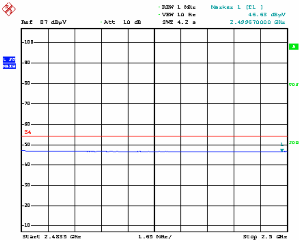
802.11n-20MHz high channel Ver AV
