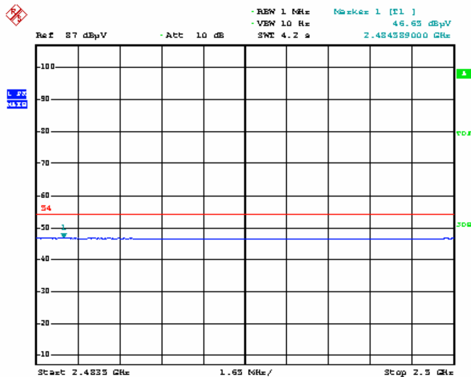
802.11n-40MHz high channel Ver AV
