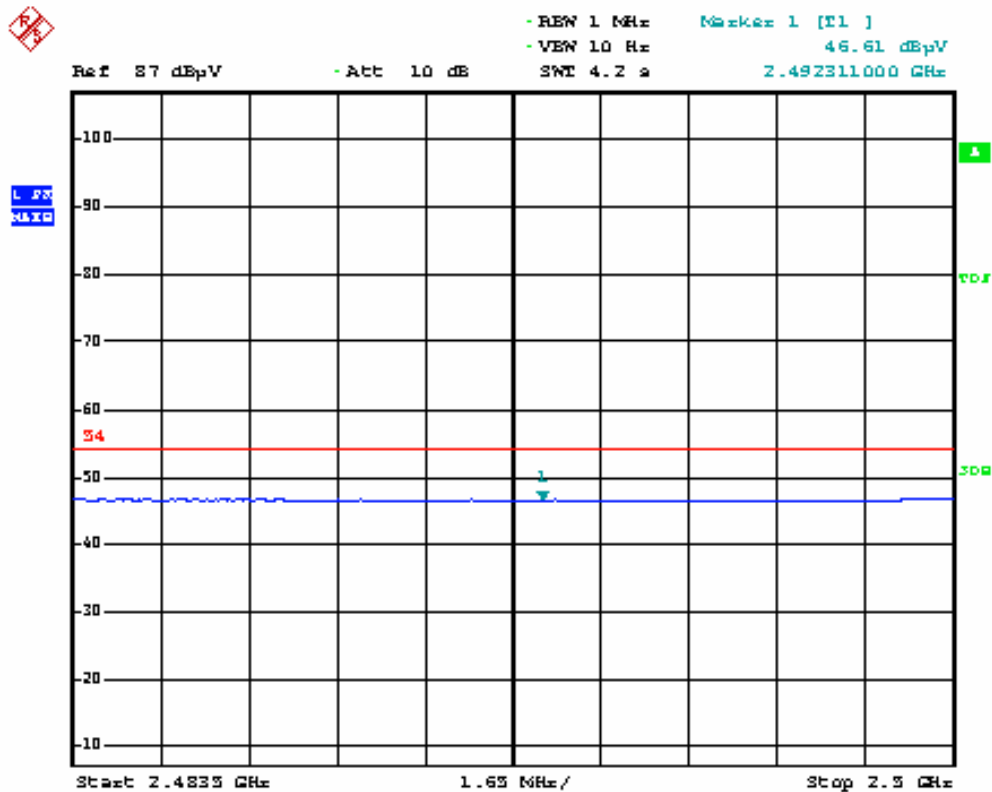
802.11n-40MHz high channel Hor AV
