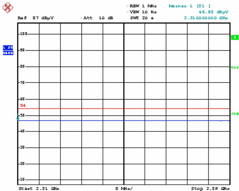
802.11b low channel Ver AV
