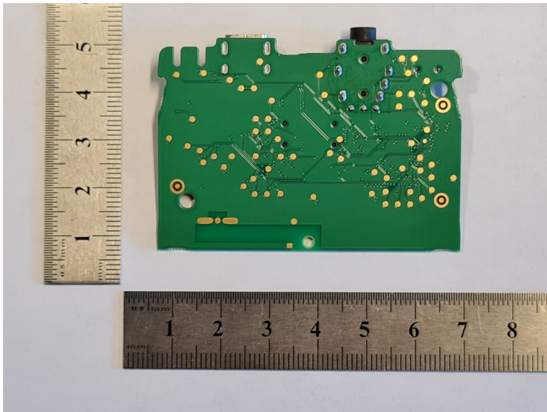
PCB-A Back
