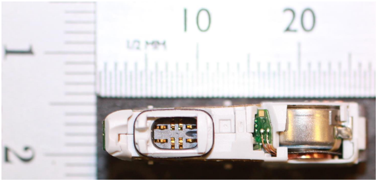
Bottom side
