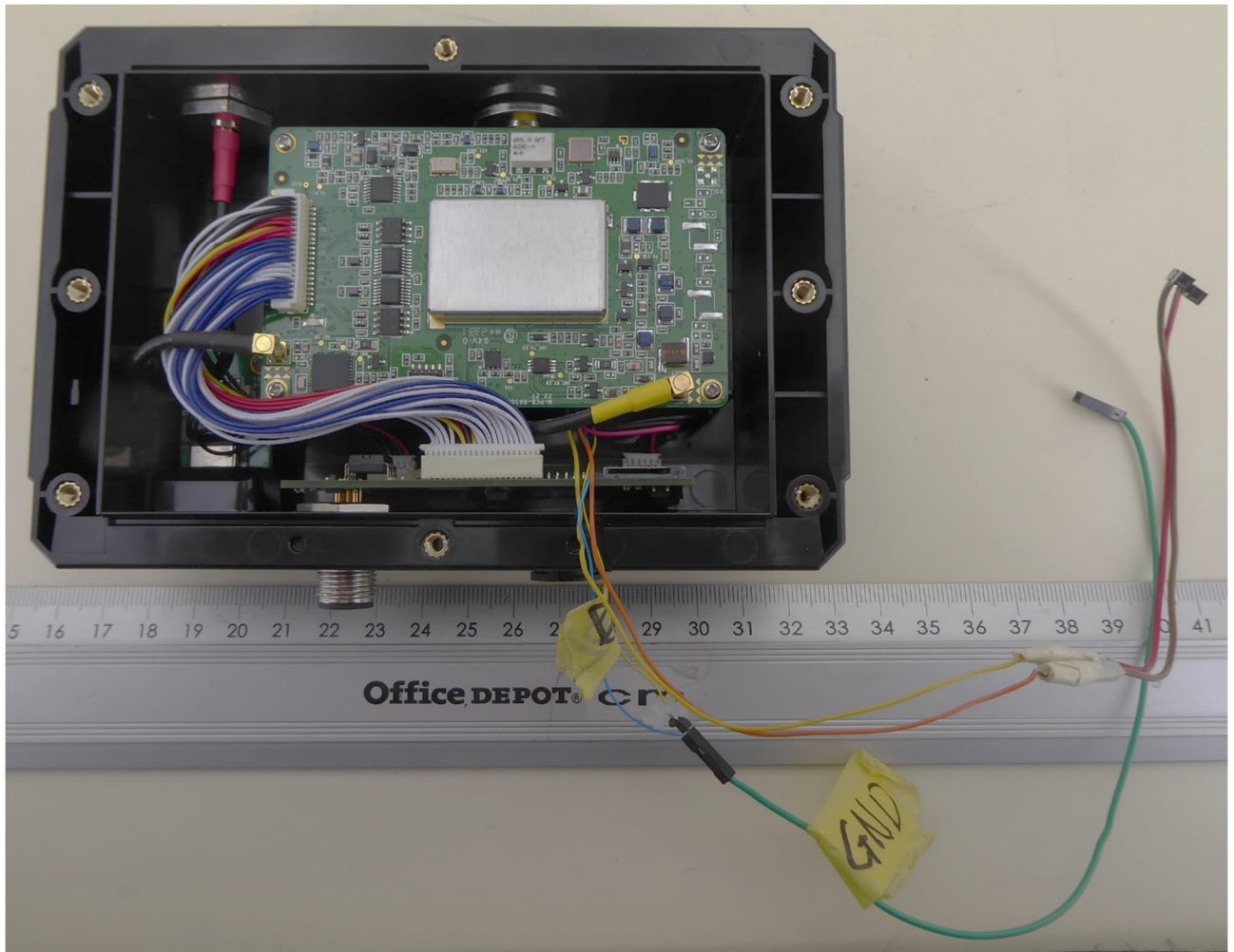
EUT open 2
