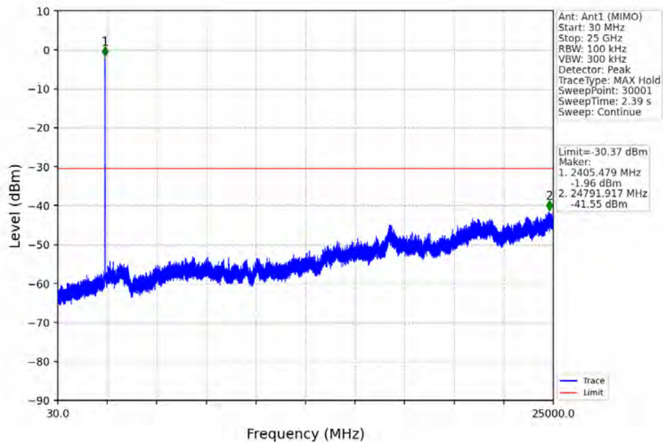
802.11g_LCH_2412MHz_Ant1 (MIMO)_NTNV
