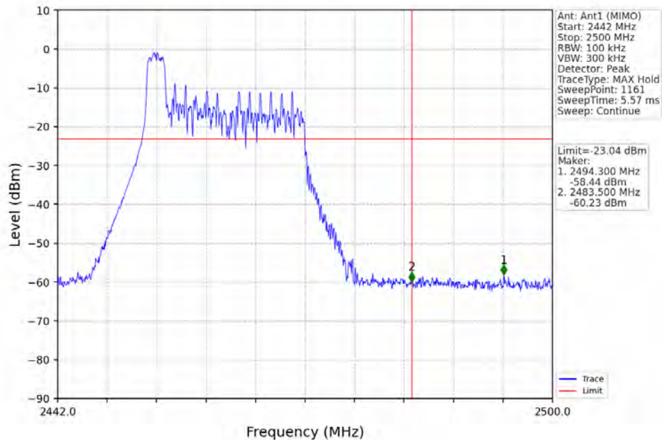
802.11ax(HEW20)_HCH_2462MHz_RU26_Left_Ant1 (MIMO)_NTNV
