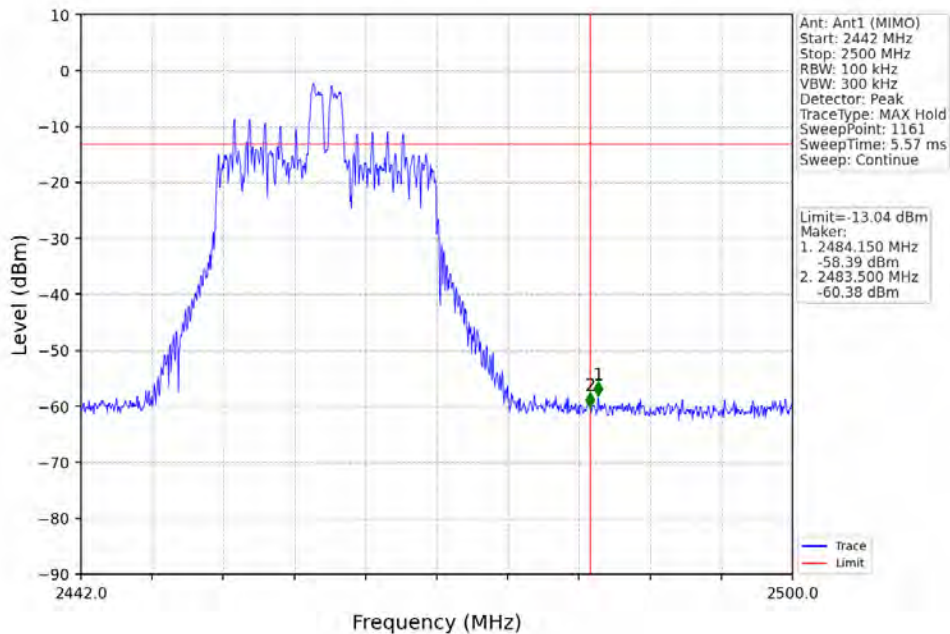
802.11ax(HEW20)_HCH_2462MHz_RU26_Mid_Ant1 (MIMO)_NTNV
