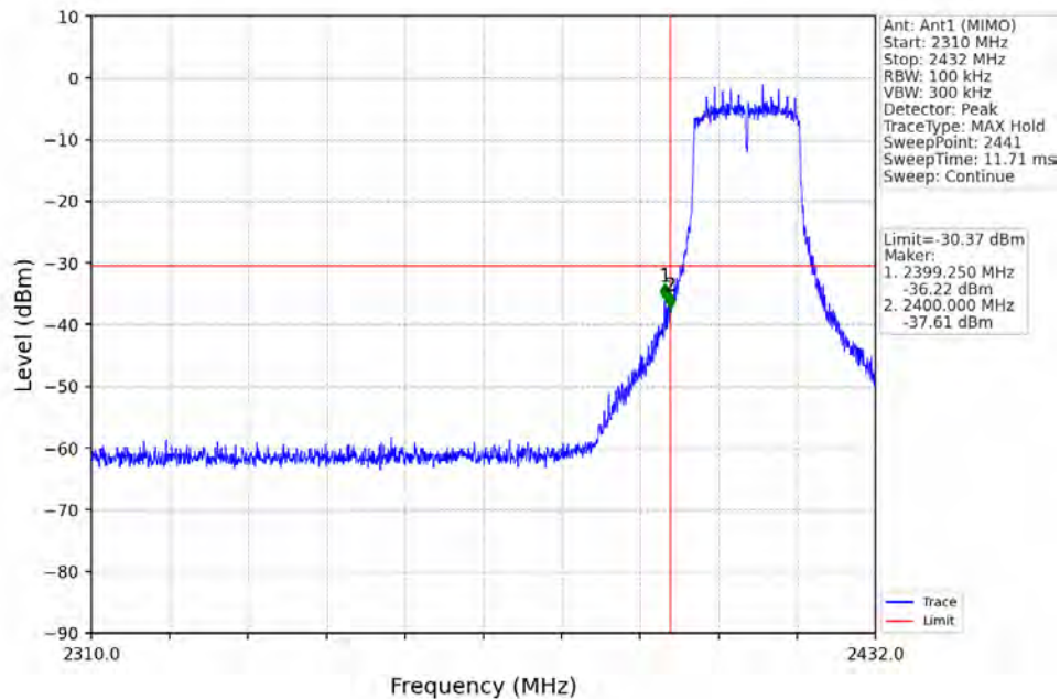
802.11g_LCH_2412MHz_Ant1 (MIMO)_NTNV
