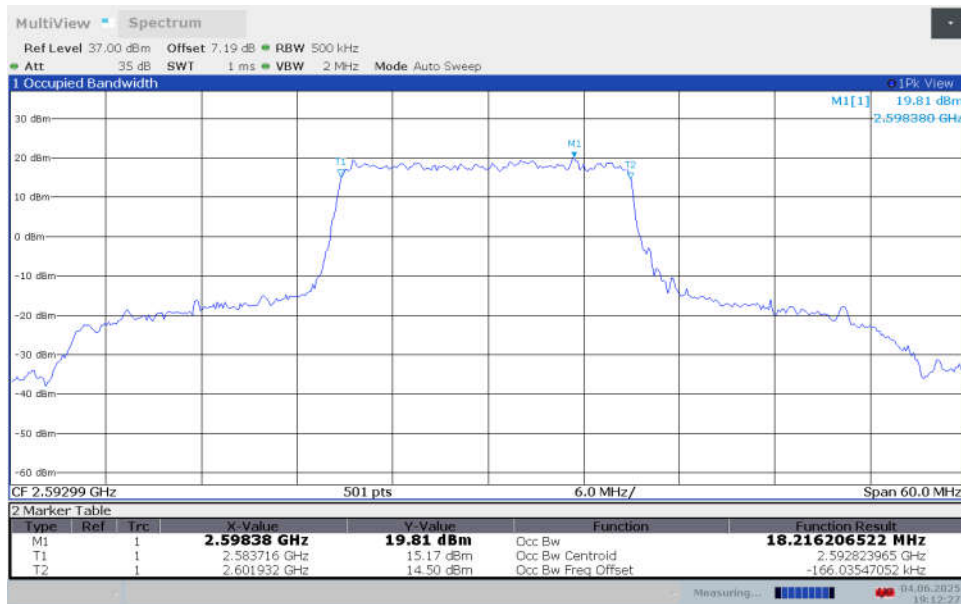
n41,20MHz Bandwidth,DFT-s-QPSK (99% BW)
