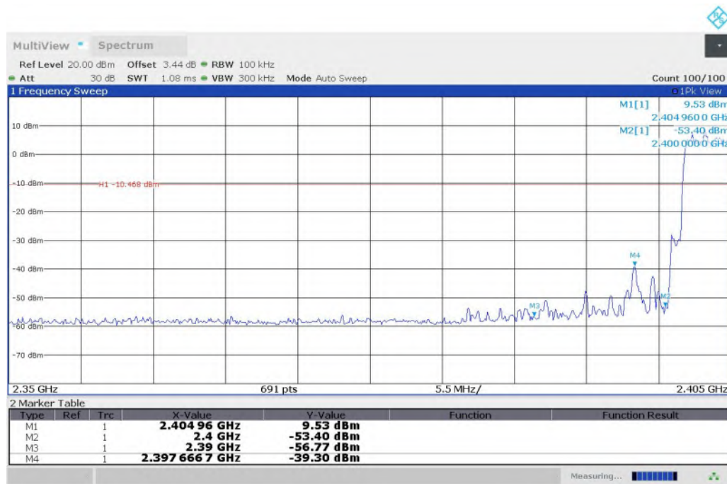
Fig. 7 Band Edges ( \pi/4 DQPSK, CH0, Hopping ON)
