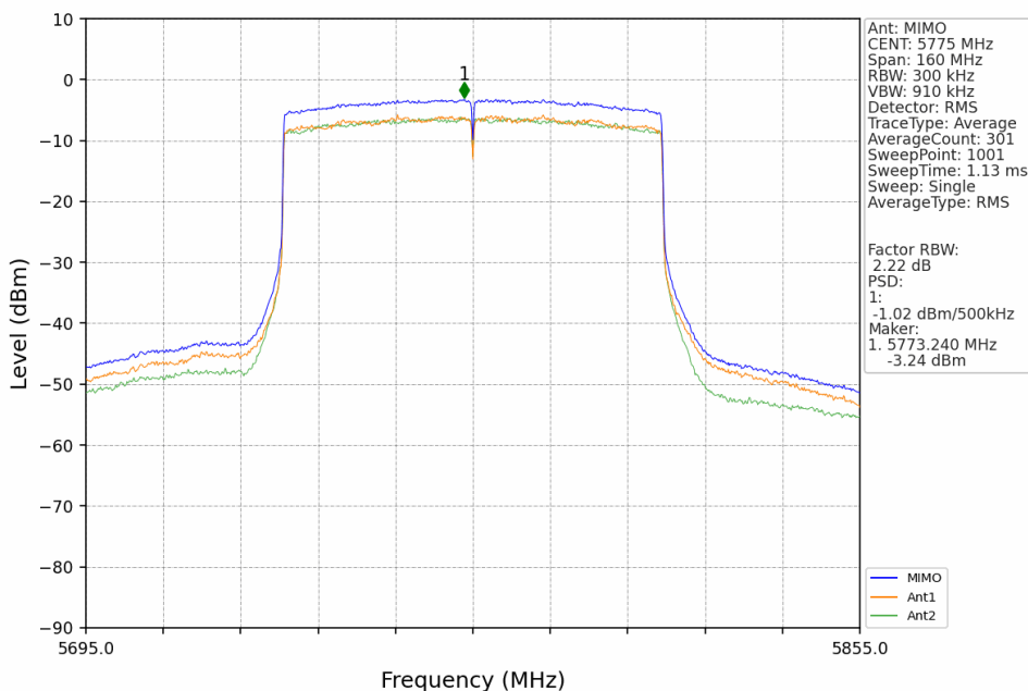
802.11ax(HEW80)_MCH_5775MHz_SU_MIMO_NTNV
