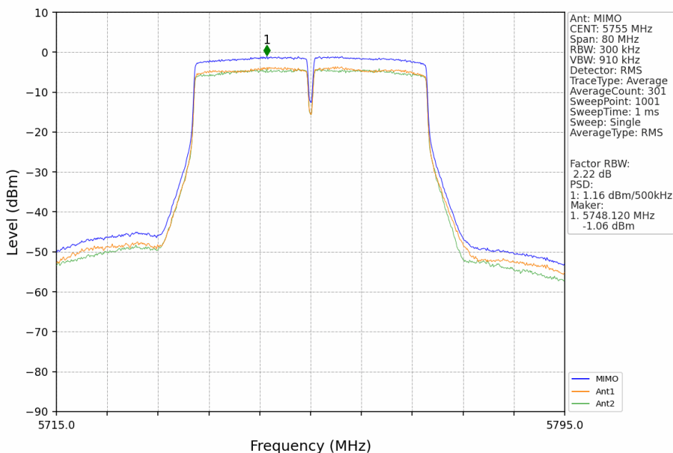
802.11ac(VHT40)_LCH_5755MHz_MIMO_NTNV
