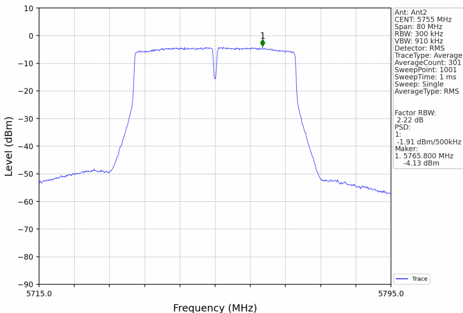
802.11ac(VHT40)_LCH_5755MHz_MIMO_NTNV
