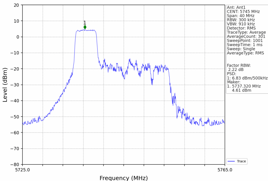
802.11ax(HEW20)_LCH_5745MHz_RU52_Left_Ant1_NTNV
