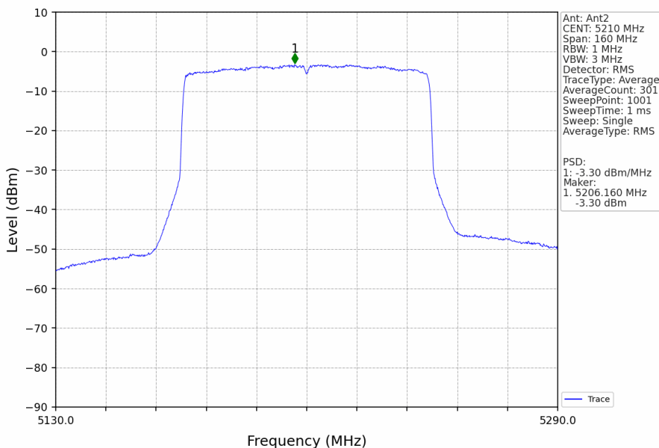
802.11ax(HEW80)_MCH_5210MHz_SU_Ant2_NTNV
