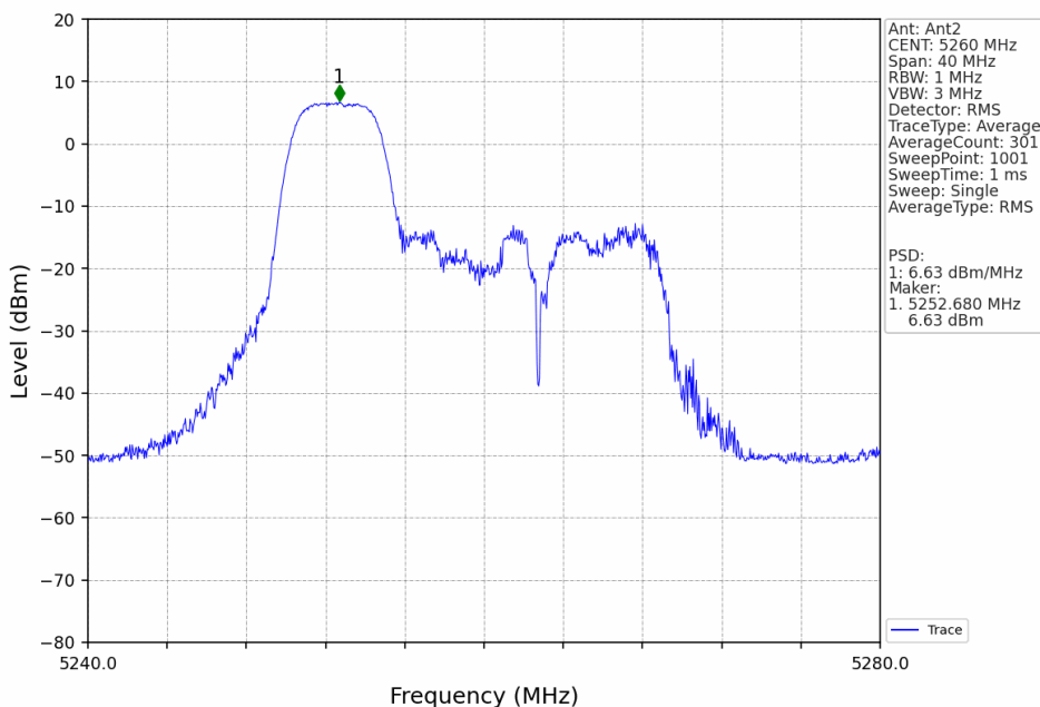
802.11ax(HEW20)_LCH_5260MHz_RU52_Left_Ant2_NTNV
