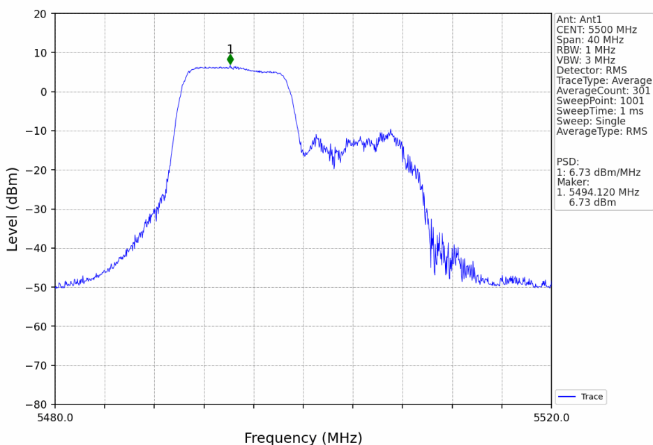
802.11ax(HEW20)_LCH_5500MHz_RU106_Left_Ant1_NTNV
