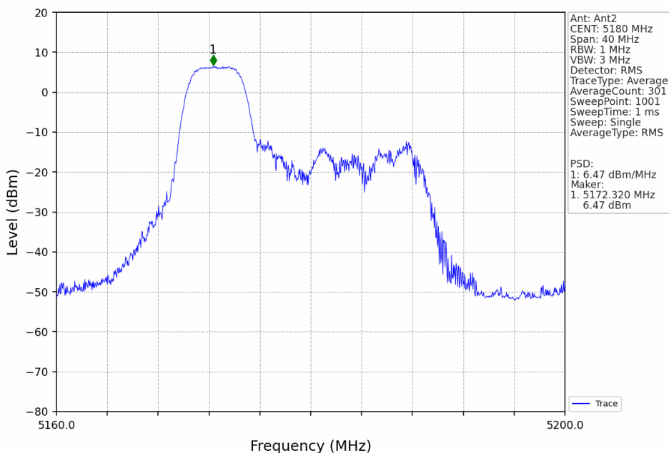
802.11ax(HEW20)_LCH_5180MHz_RU52_Left_Ant2_NTNV
