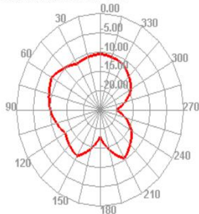
3500.000MHz E1
