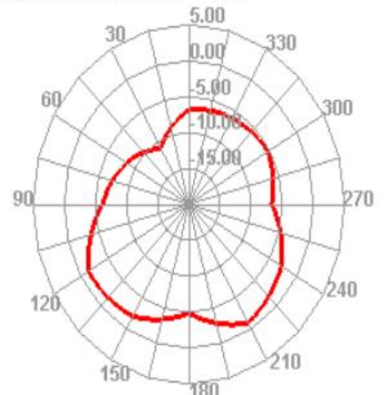
1900.000MHz E2
