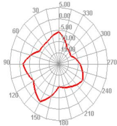
2500.000MHz E1
