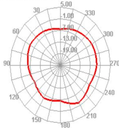
2500.000MHz H
