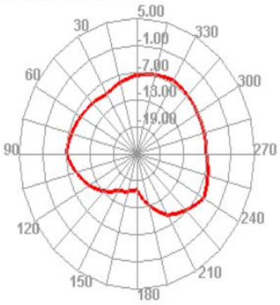
2600.000MHz H
