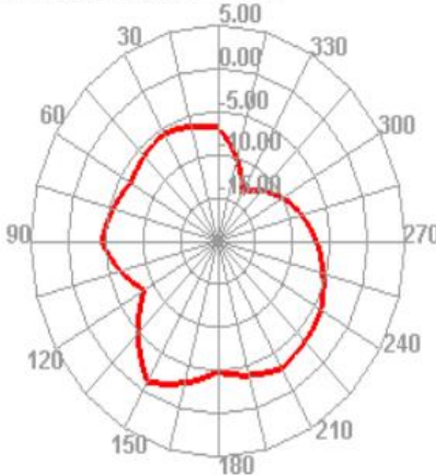
1900.000MHz E1
