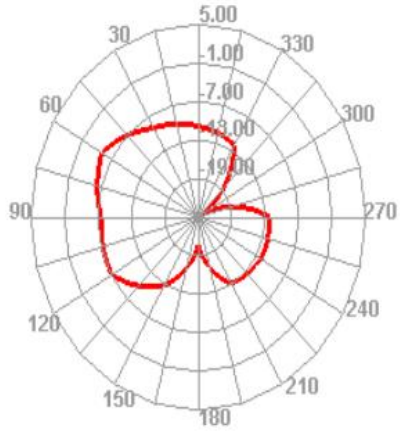
4200.000MHz H
