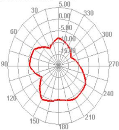
1800.000MHz E1
