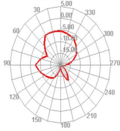
2600.000MHz E1
