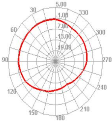
2500.000MHz H
