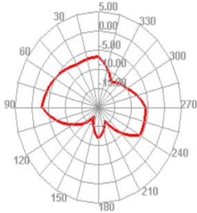
5500.000MHz E1
