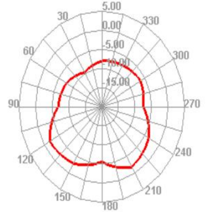
1800.000MHz E2
