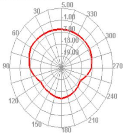
1800.000MHz H
