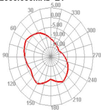
2350.000MHz E1
