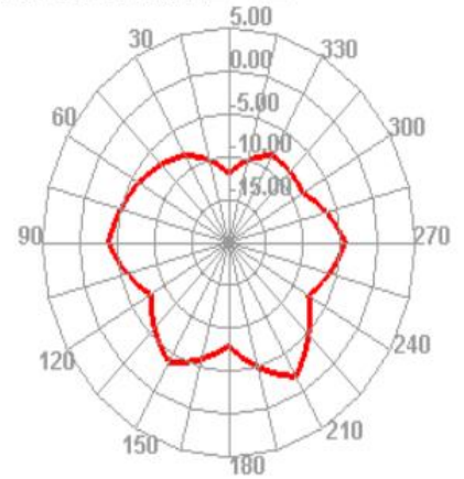
2600.000MHz E2
