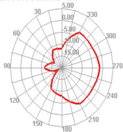
2600.000MHz E1
