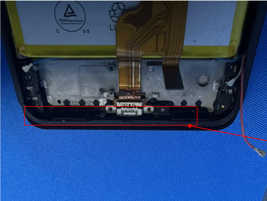
Ant4
