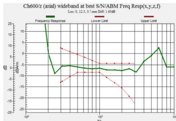
Fig 7.2 CDMA2000 BC1 Ch600
