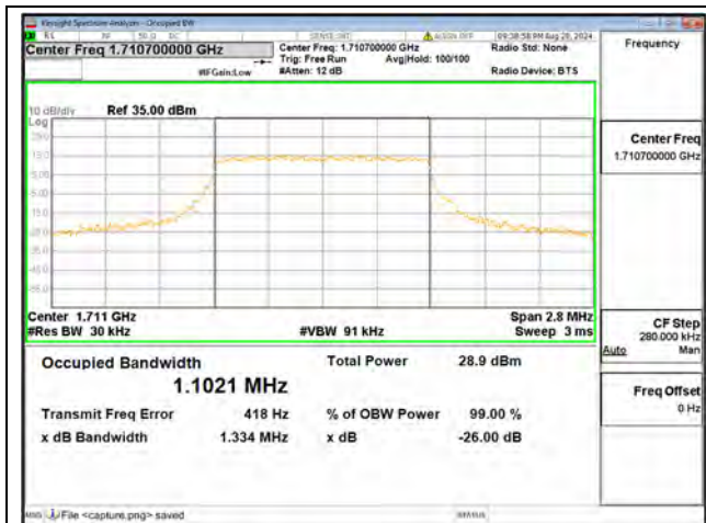
B66 / 1.4MHz / QPSK / Low CH
