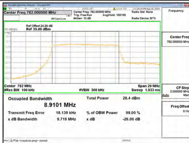
B13 / 10MHz / 64QAM / Mid CH
