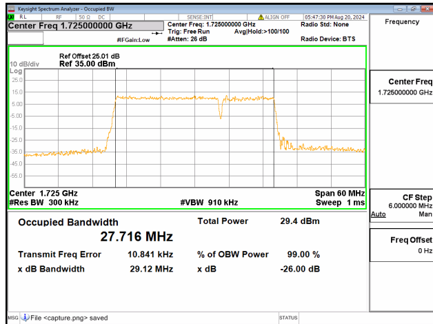
66C / 20+10MHz / 64QAM/ Low CH
