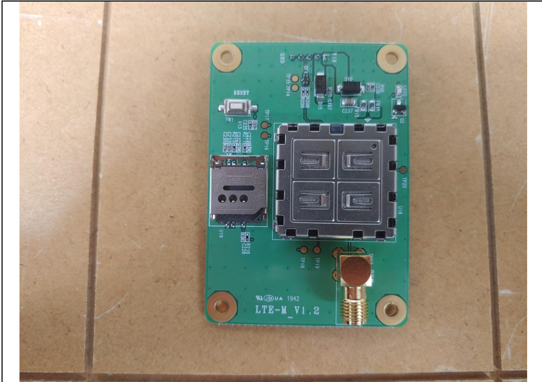
WCDMA module Front
