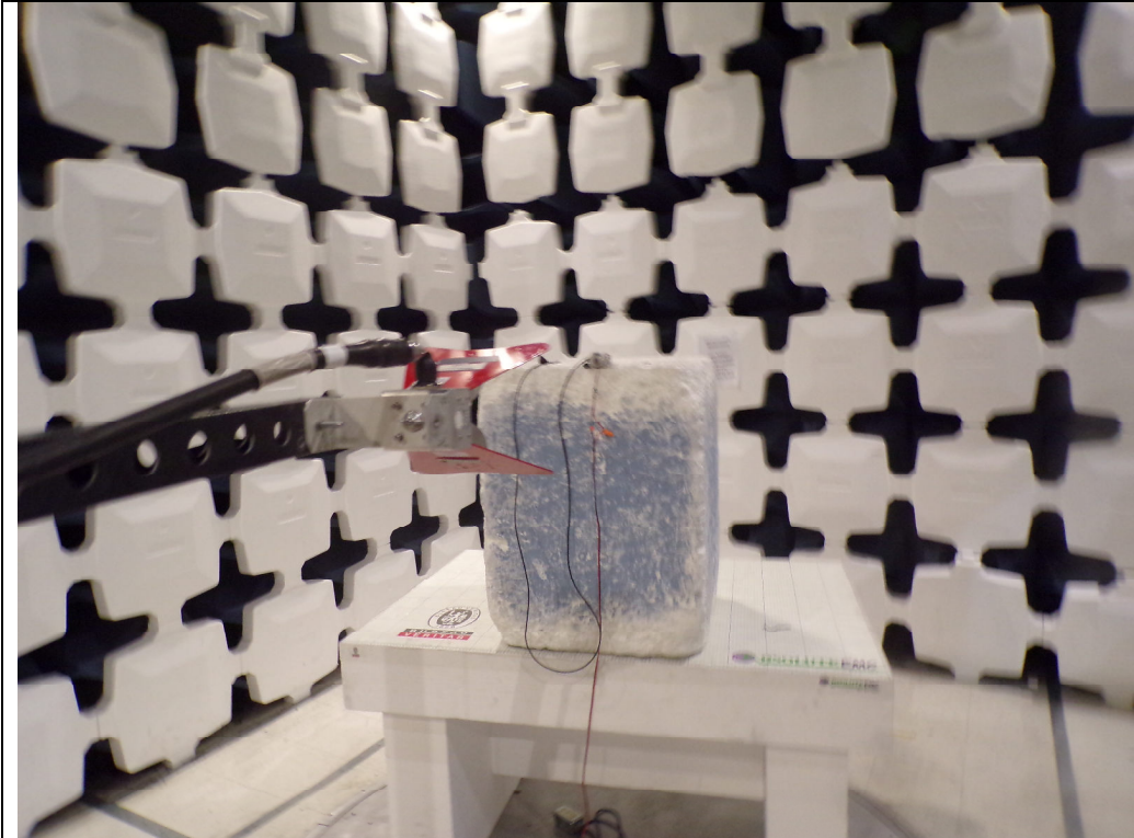
6GHz-18GHz
