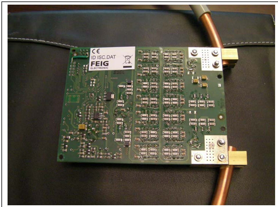
FEIG DAT Board in Wand Bottom
