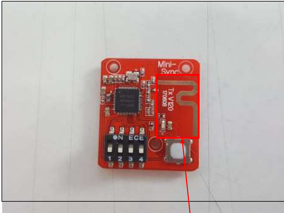
PIFA Antenna
