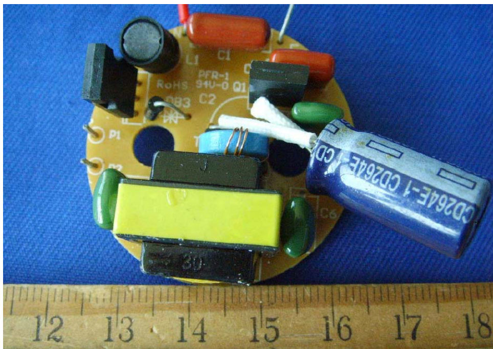
EUT –Components View (HLFR23W)
