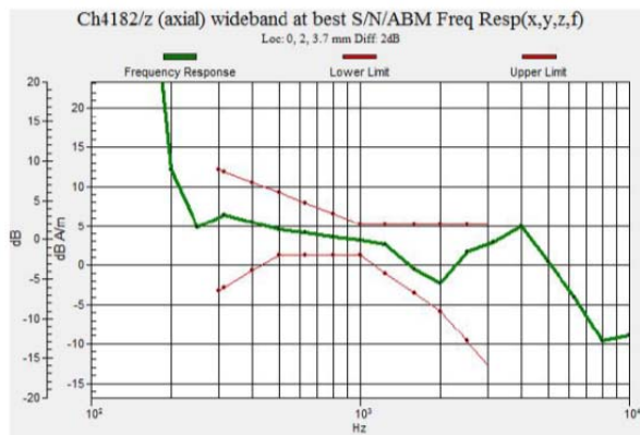
Fig. 9.3 WCDMA Band V Ch4182
