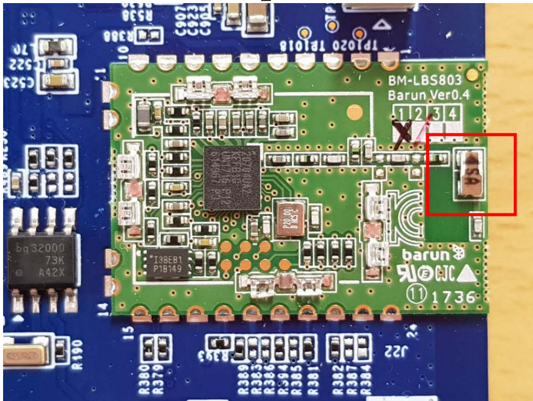
BT/BLE_Antenn
