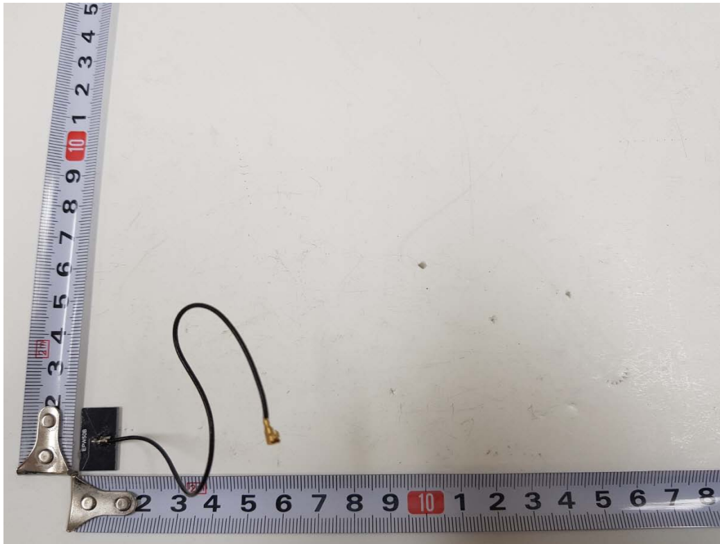
WLAN 5GHz_Antenna
