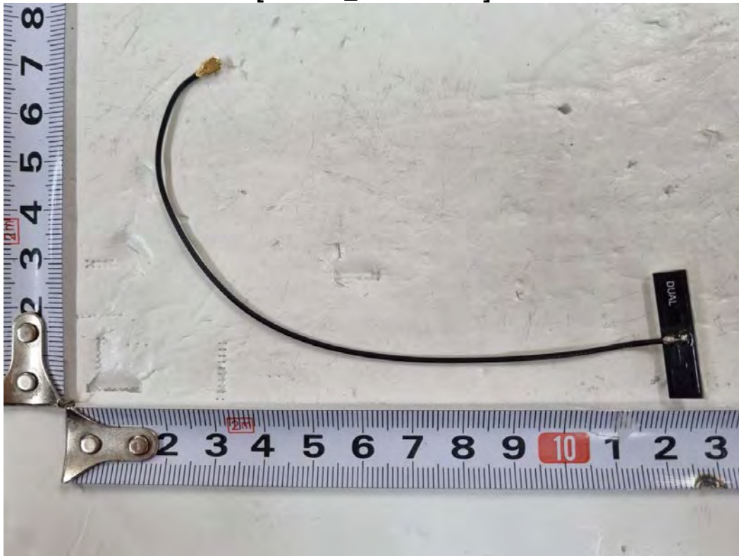
[WLAN_Antenna3]
