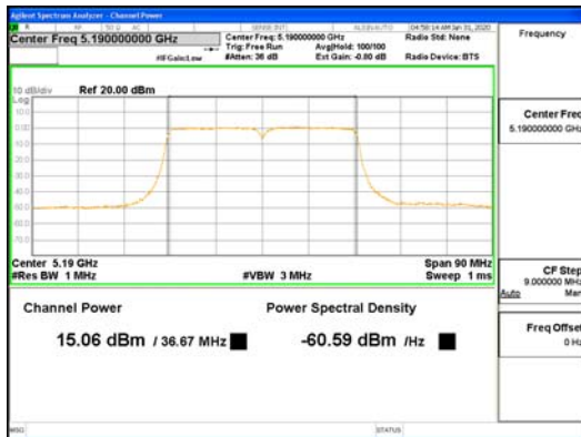
SDM Mode ANT1 802.11ac VHT40 UNII-1
