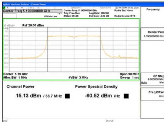
CDD Mode ANT1 802.11ac VHT40 UNII-1
