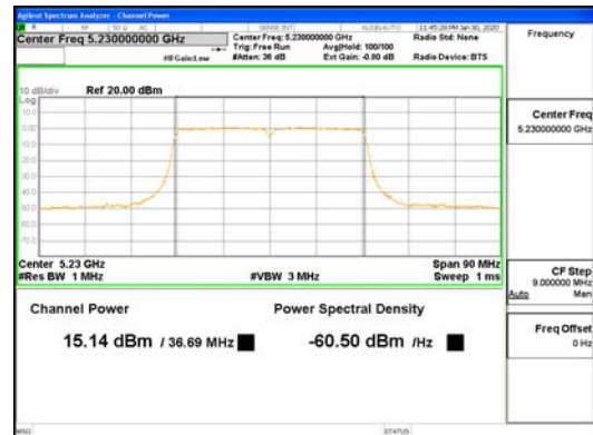
CDD Mode ANT1 802.11ac VHT40 UNII-1
