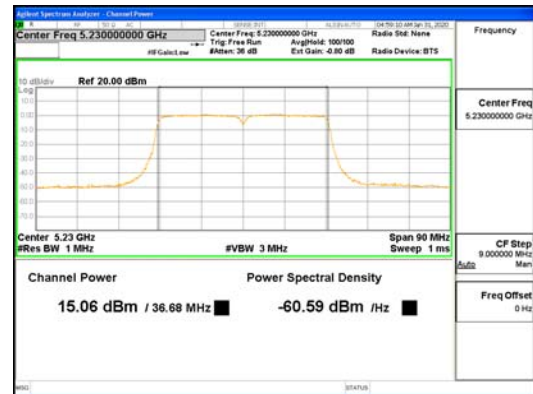
SDM Mode ANT1 802.11ac VHT40 UNII-1
