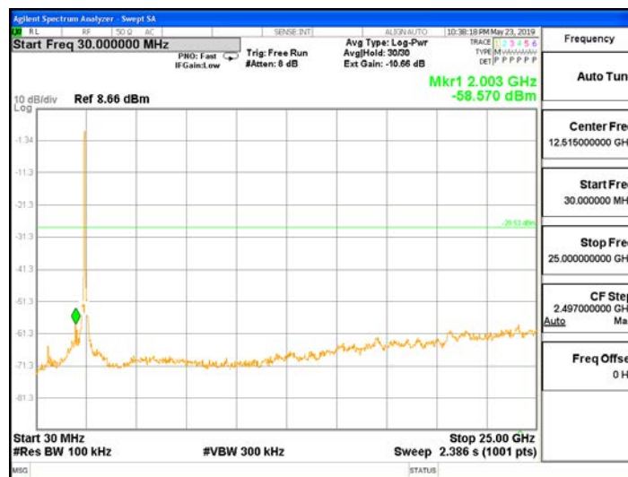
802.11n_HT40_ANT1
