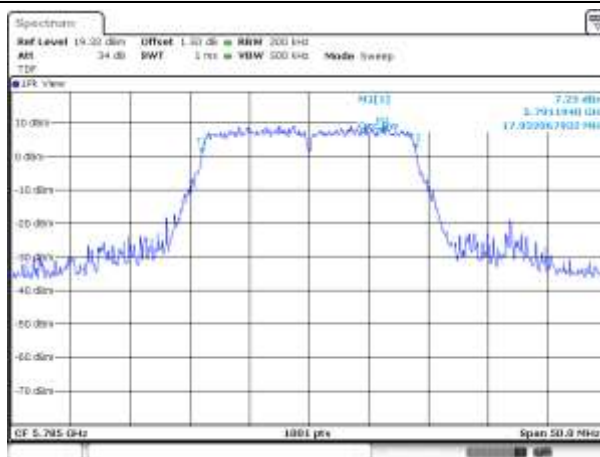
UNII-3 / 802.11ac VHT20 / 5 785 MHz
