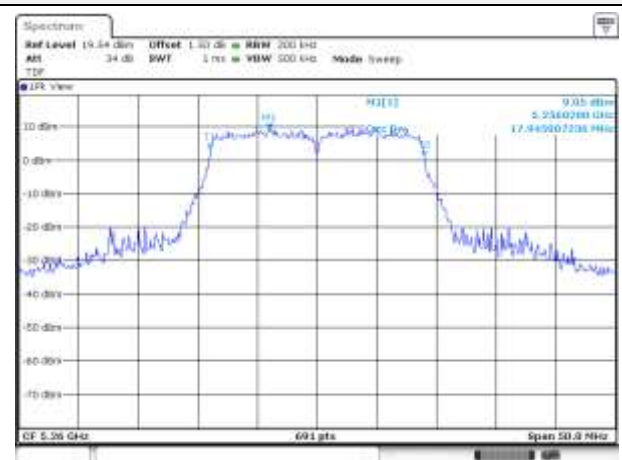
UNII-2A / 802.11ac VHT20 / 5 260 MHz
