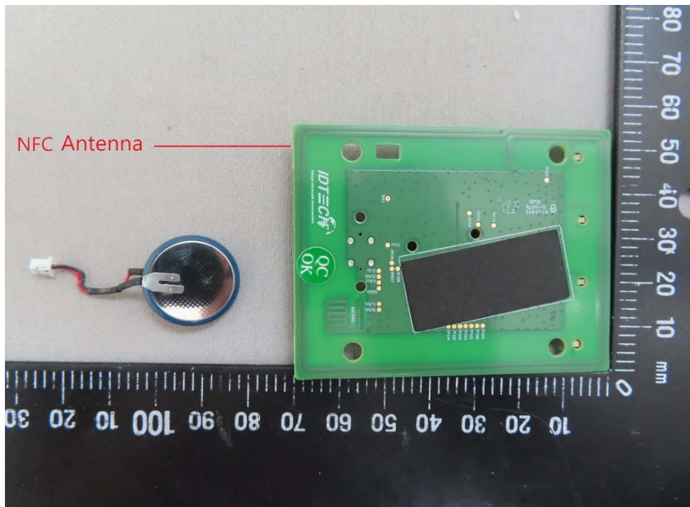
NFC Antenna
