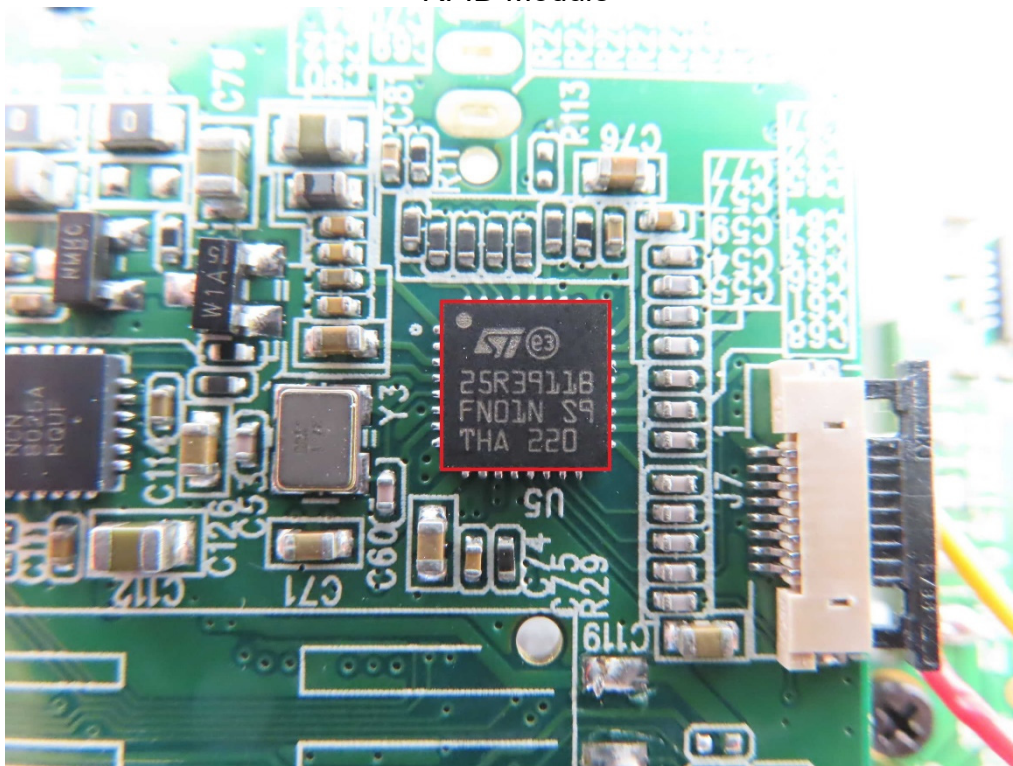
RFID Module
