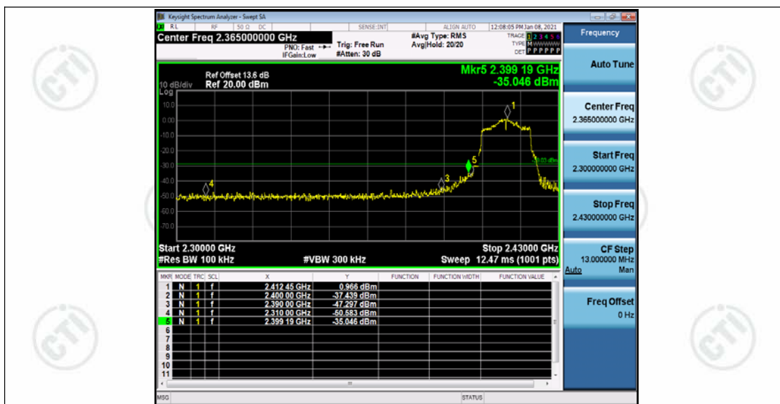
11G_Ant1_Low_2412
