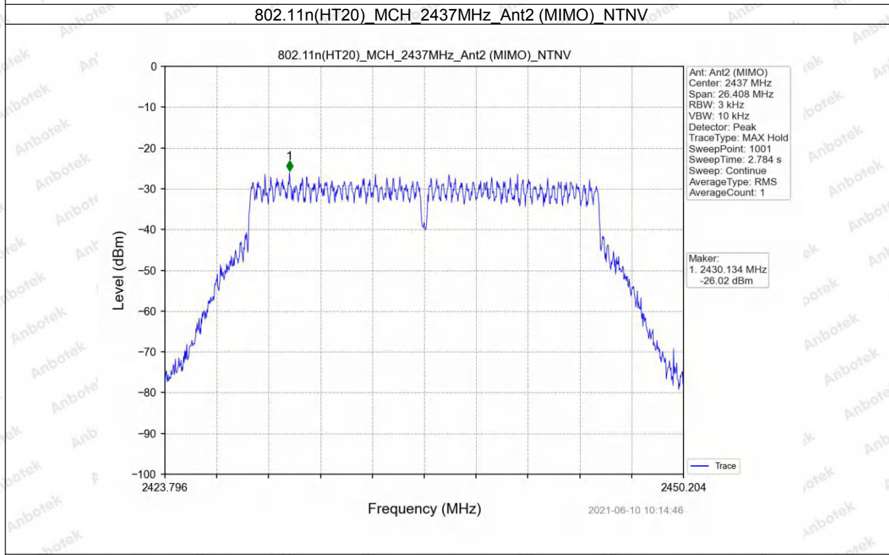
802.11n(HT20)_MCH_2437MHz_MIMO_NTNV
