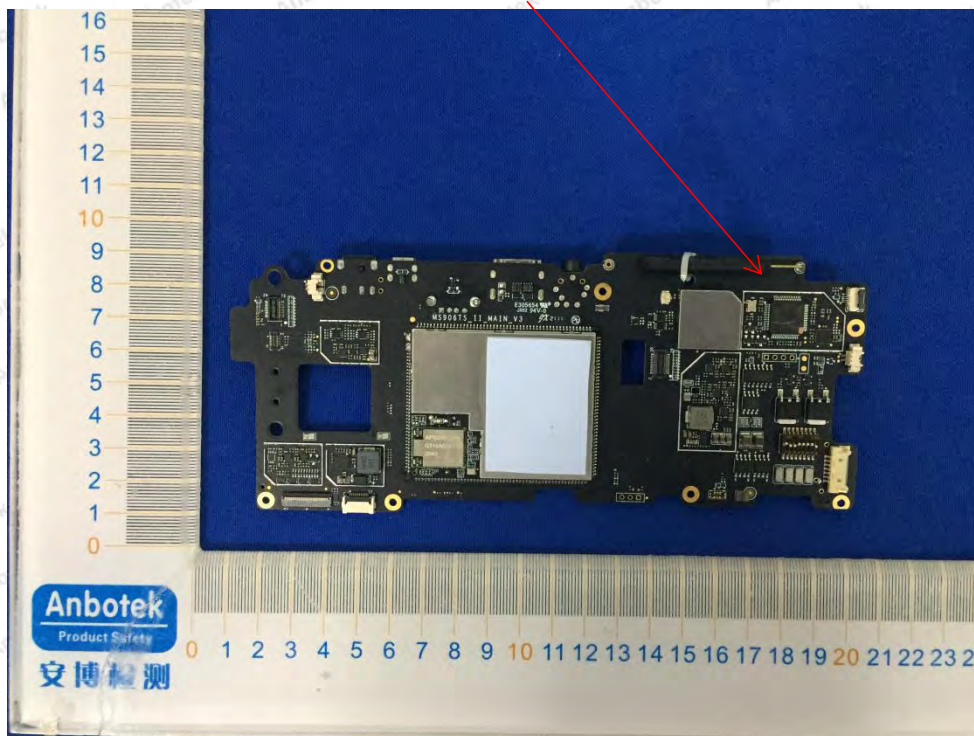
315MHz&433.92MHz&125KHz ANT
