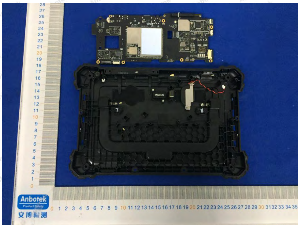
315MHz&433.92MHz&125KHz ANT
