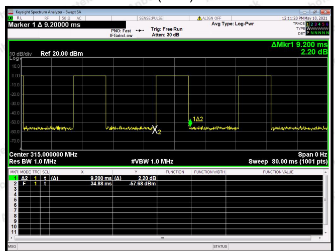
315MHz(FSK)-T on1
