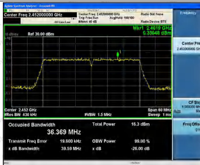
11N40 Ant2 2452
