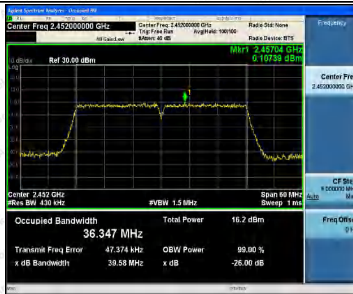
11N40 Ant2 2452
