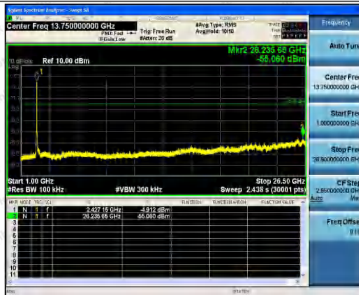
11N40_Ant2_2422_1000~26500
