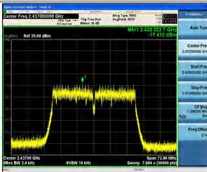
11N40_Ant2_2437
