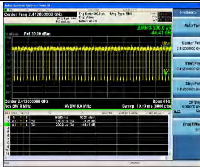
11N20_Ant2_2412
