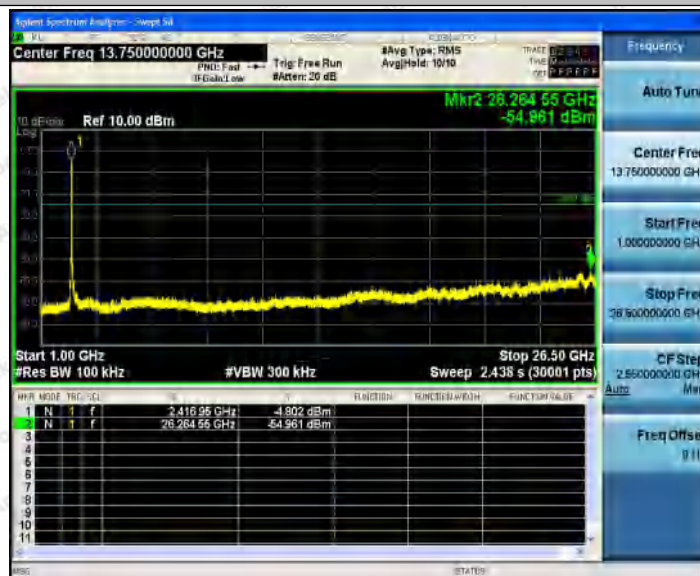
11N40_Ant2_2422_0~Reference
