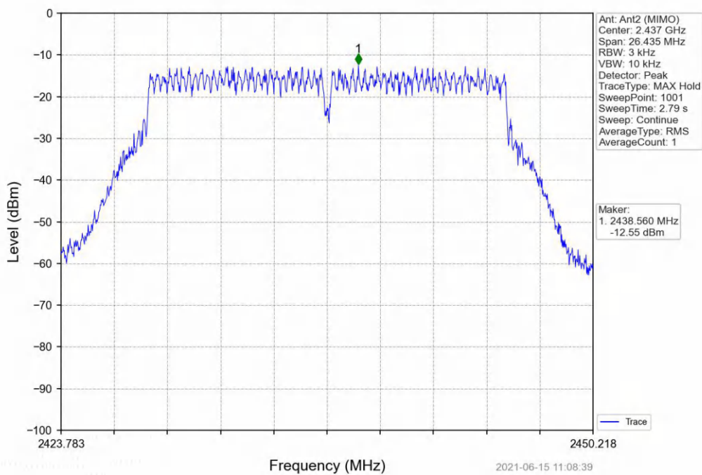
802.11n(HT20)_MCH_2437MHz_MIMO_NTNV
