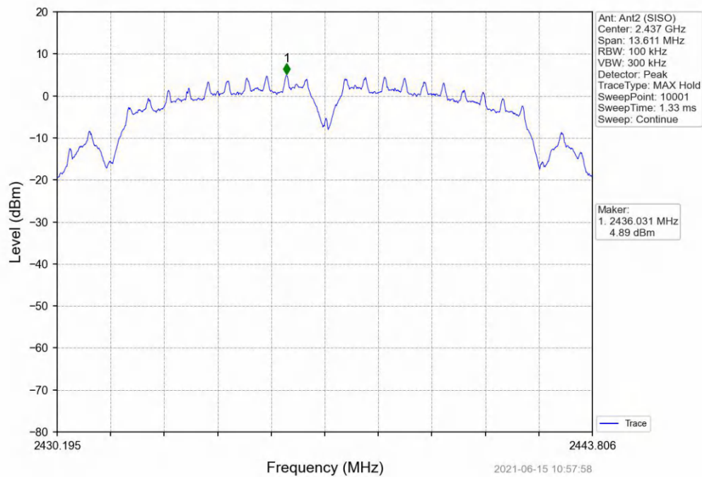
802.11b_MCH_2437MHz_Ant2 (SISO)_NTNV
