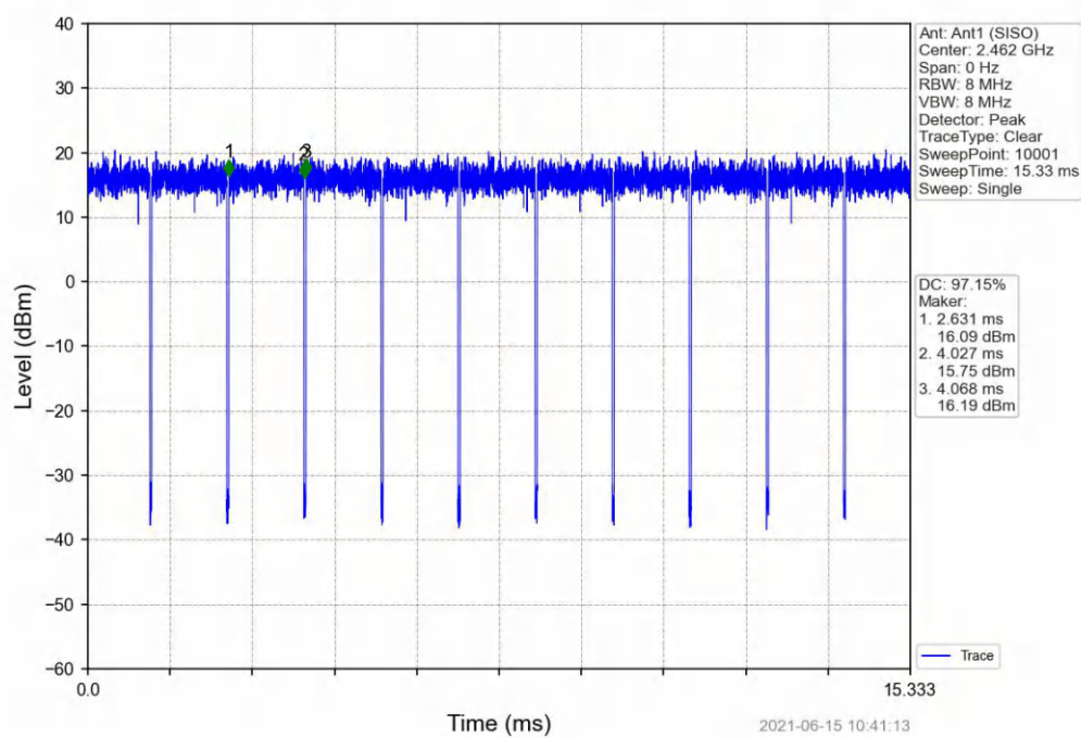
802.11g_HCH_2462MHz_Ant1 (SISO)_NTNV
