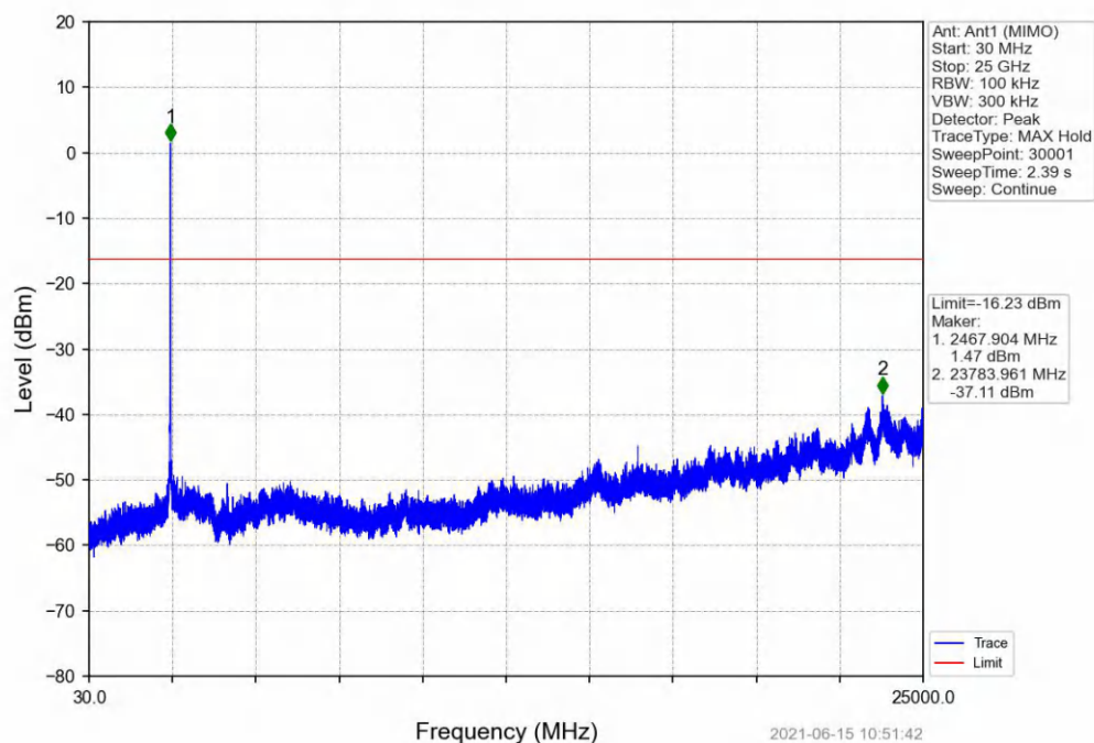
802.11n(HT20)_HCH_2462MHz_Ant1 (MIMO)_NTNV
