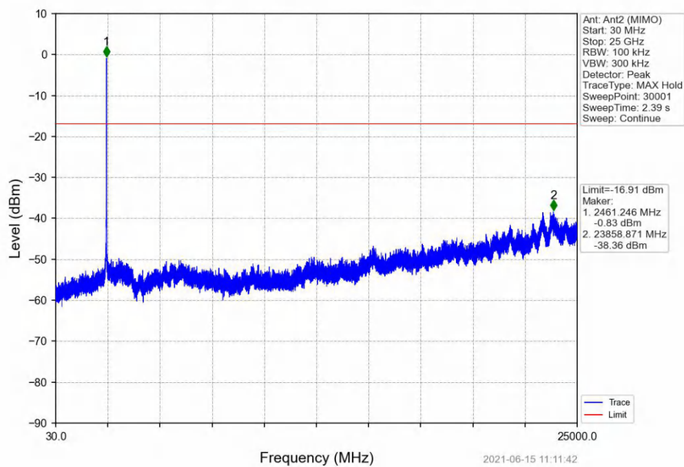
802.11n(HT20)_HCH_2462MHz_Ant2 (MIMO)_NTNV
