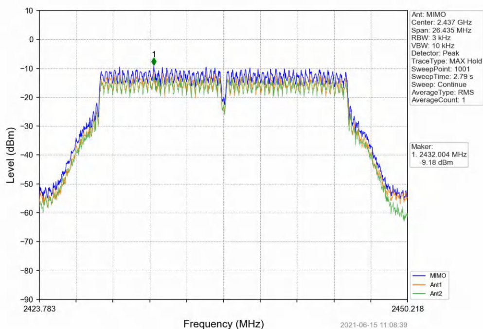
802.11n(HT20)_MCH_2437MHz_MIMO_NTNV
