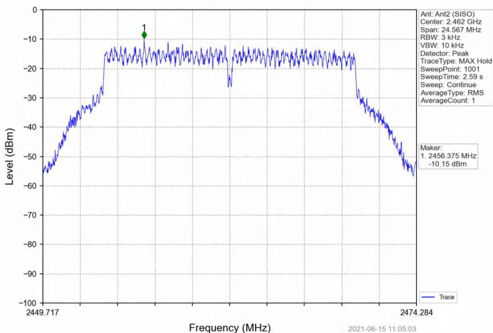
802.11g_HCH_2462MHz_Ant2 (SISO)_NTNV
