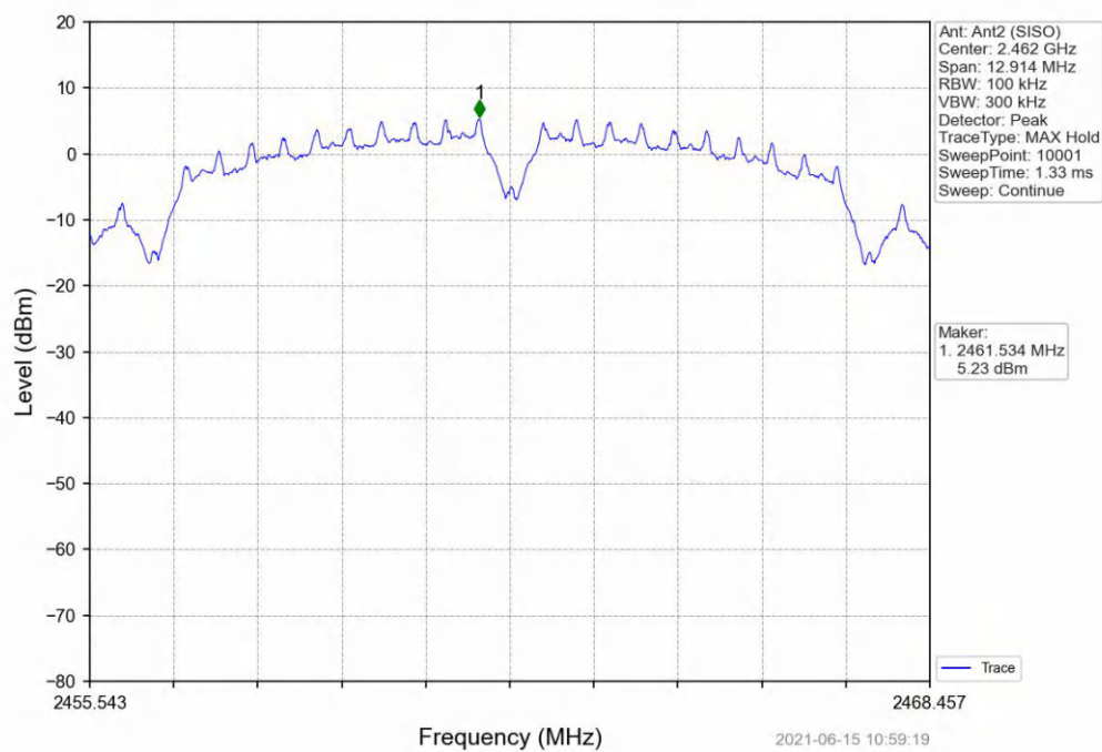
802.11b_HCH_2462MHz_Ant2 (SISO)_NTNV
