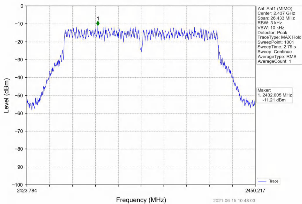
802.11n(HT20)_MCH_2437MHz_Ant1 (MIMO)_NTNV
