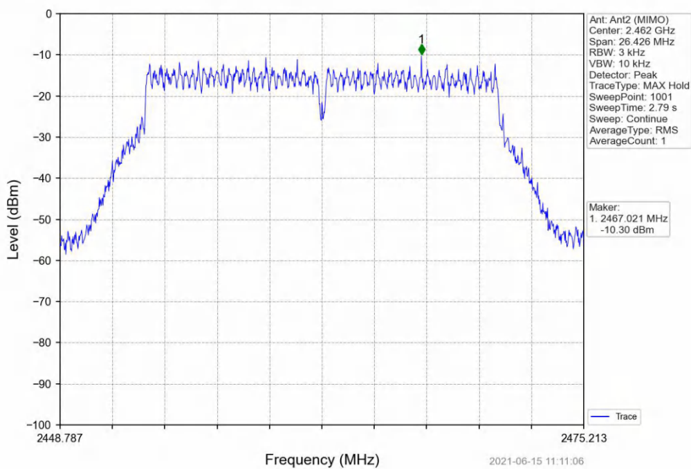
802.11n(HT20)_HCH_2462MHz_Ant2 (MIMO)_NTNV
