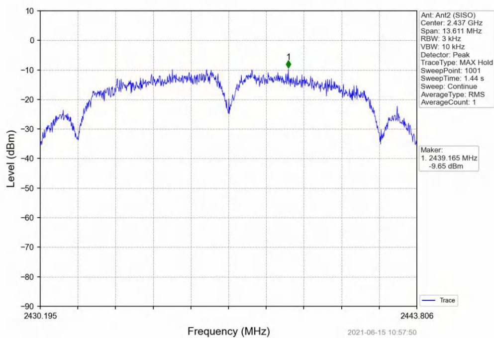
802.11b_MCH_2437MHz_Ant2 (SISO)_NTNV
