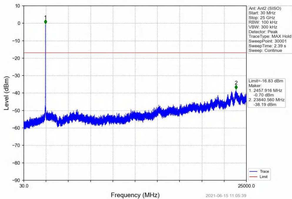
802.11g_HCH_2462MHz_Ant2 (SISO)_NTNV
