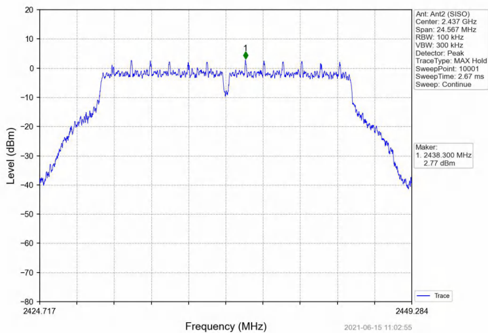
802.11g_MCH_2437MHz_Ant2 (SISO)_NTNV
