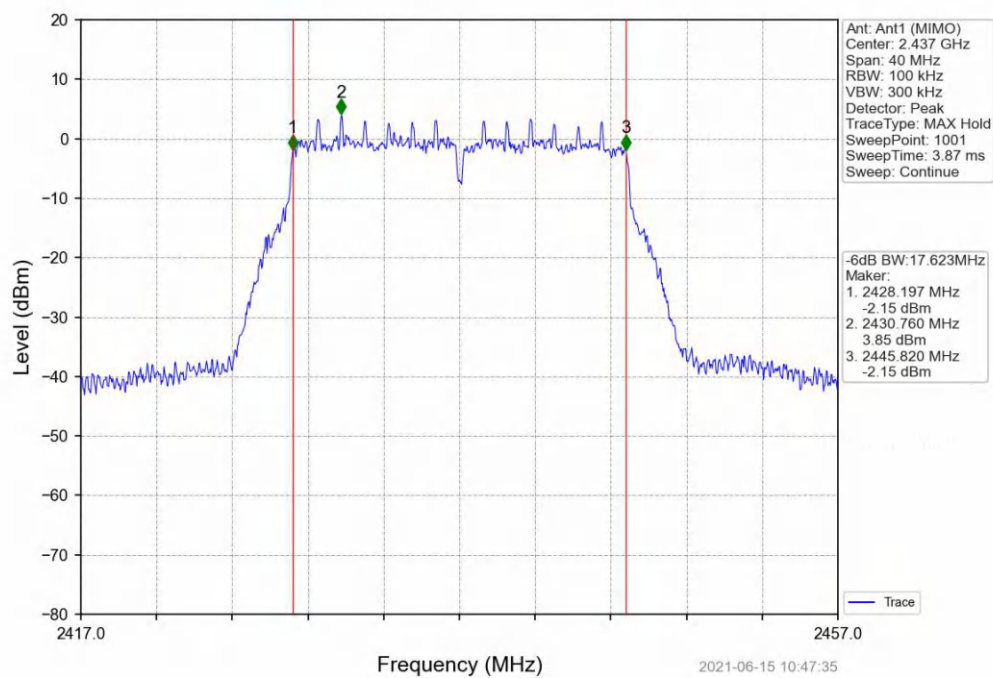
802.11n(HT20)_MCH_2437MHz_Ant1 (MIMO)_NTNV
