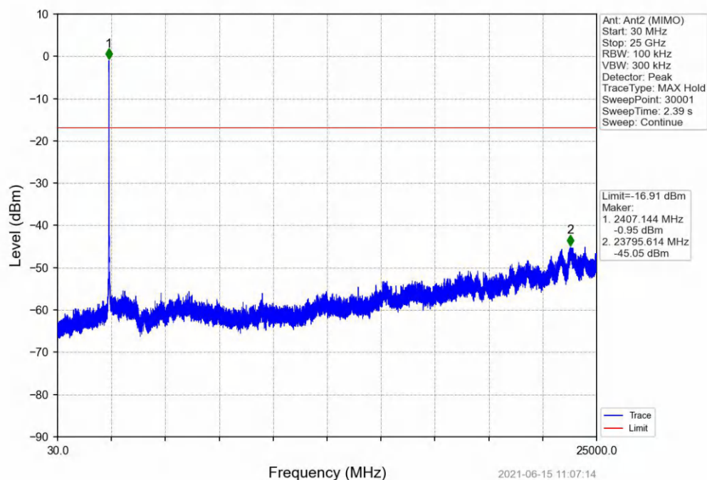
802.11n(HT20)_LCH_2412MHz_Ant2 (MIMO)_NTNV
