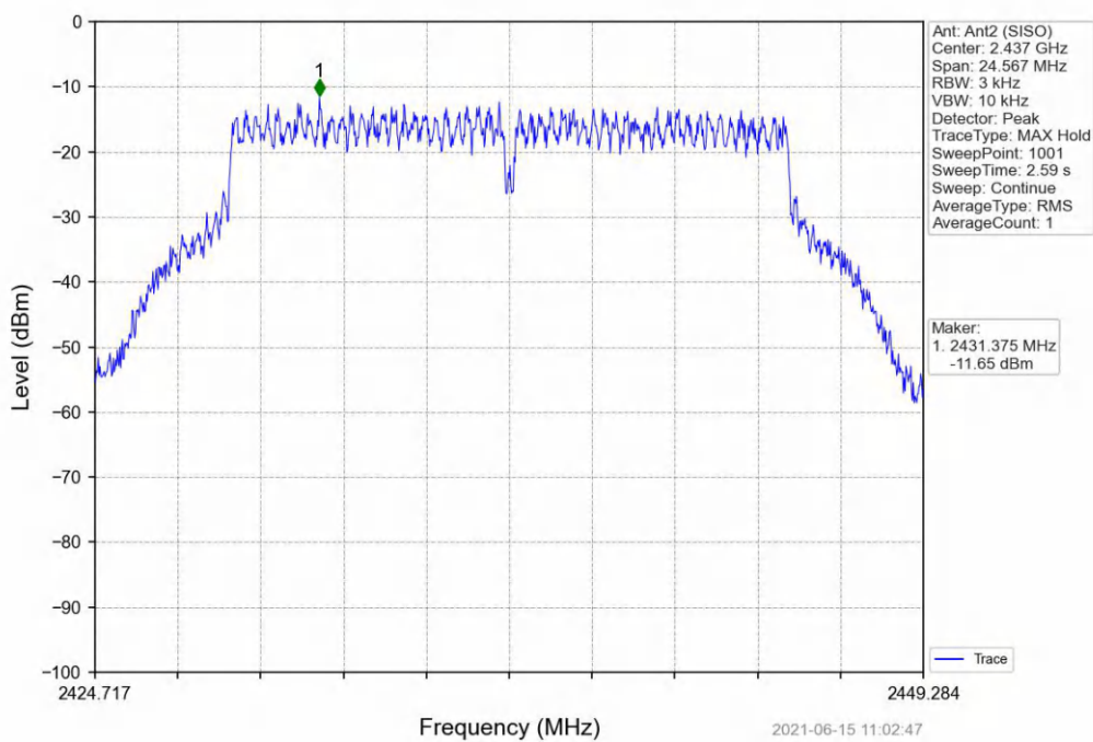
802.11g_MCH_2437MHz_Ant2 (SISO)_NTNV
