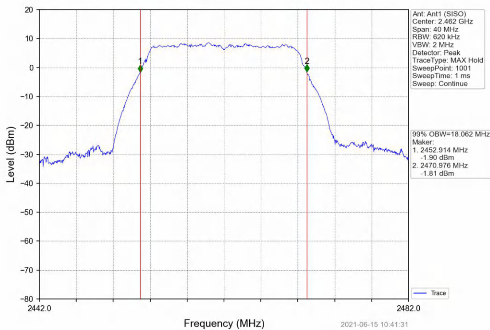
802.11g_HCH_2462MHz_Ant1 (SISO)_NTNV
