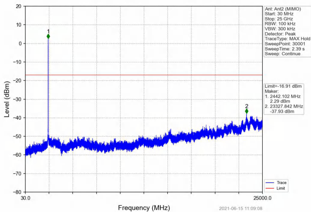
802.11n(HT20)_MCH_2437MHz_Ant2 (MIMO)_NTNV
