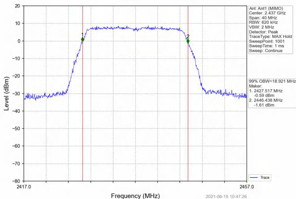
802.11n(HT20)_MCH_2437MHz_Ant1 (MIMO)_NTNV
