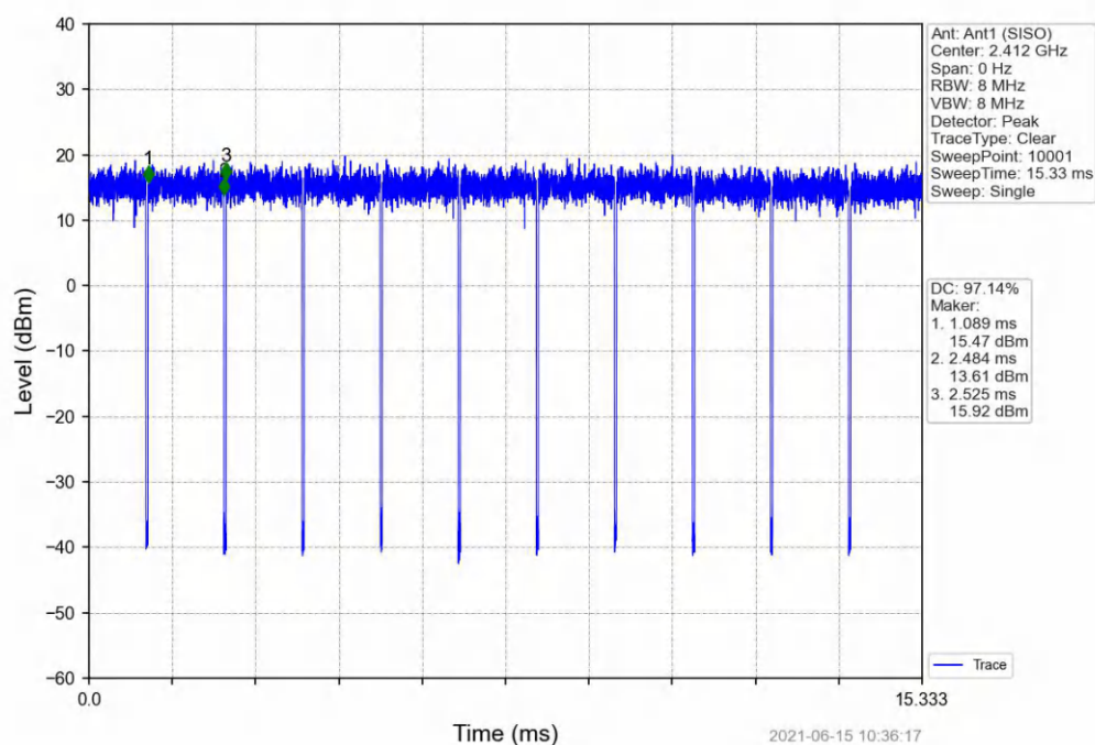
802.11g_LCH_2412MHz_Ant1 (SISO)_NTNV
