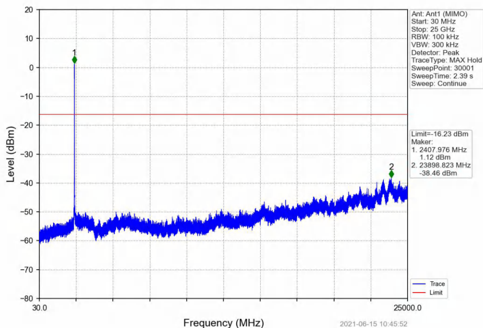
802.11n(HT20)_LCH_2412MHz_Ant1 (MIMO)_NTNV
