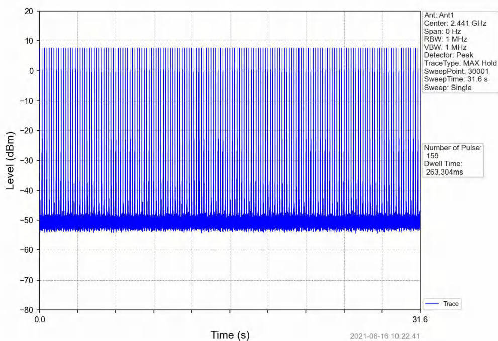
GFSK_DH3_HOPP_Ant1_NTNV
