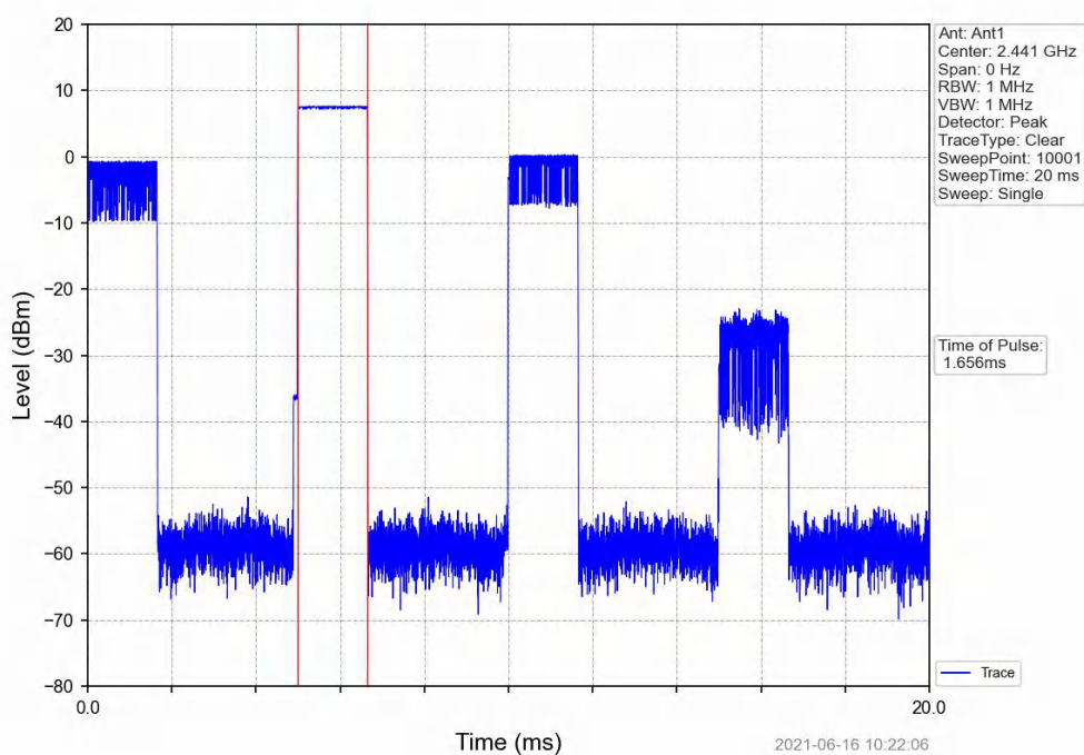
GFSK_DH3_HOPP_Ant1_NTNV
