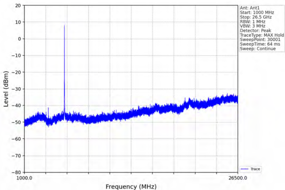
802.11a MCH_5785MHz_Ant1_NTNV
