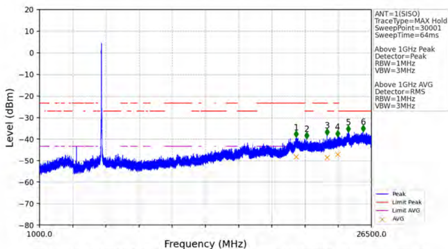
802.11n(HT40)_LCH_5755MHz_Ant1_NTNV
