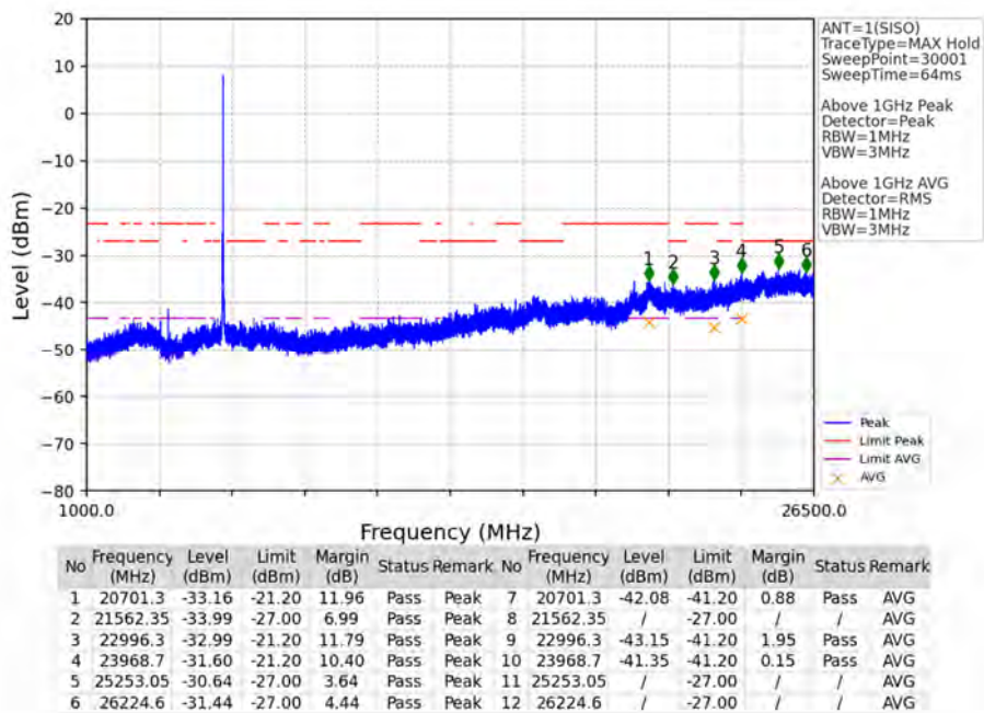
802.11a MCH_5785MHz_Ant1_NTNV
