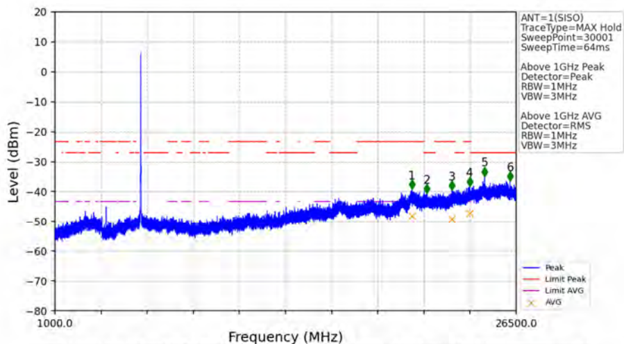
802.11n(HT20)_LCH_5745MHz_Ant1_NTNV
