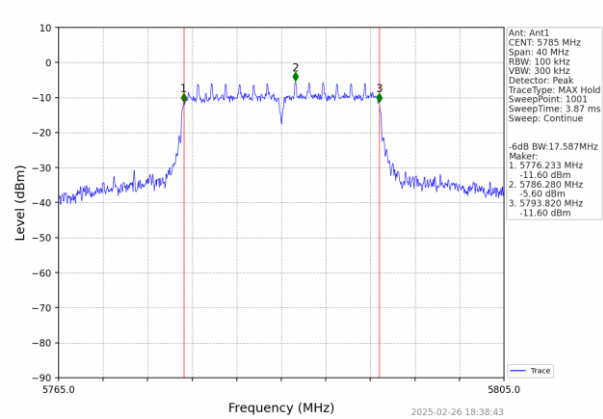
802.11n(HT20)_MCH_5785MHz_Ant1_NTNV
