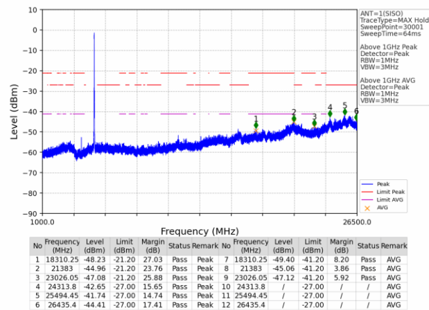
802.11a_MCH_5200MHz_Ant1_NTNV
