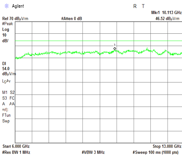
EUT Ant.2
