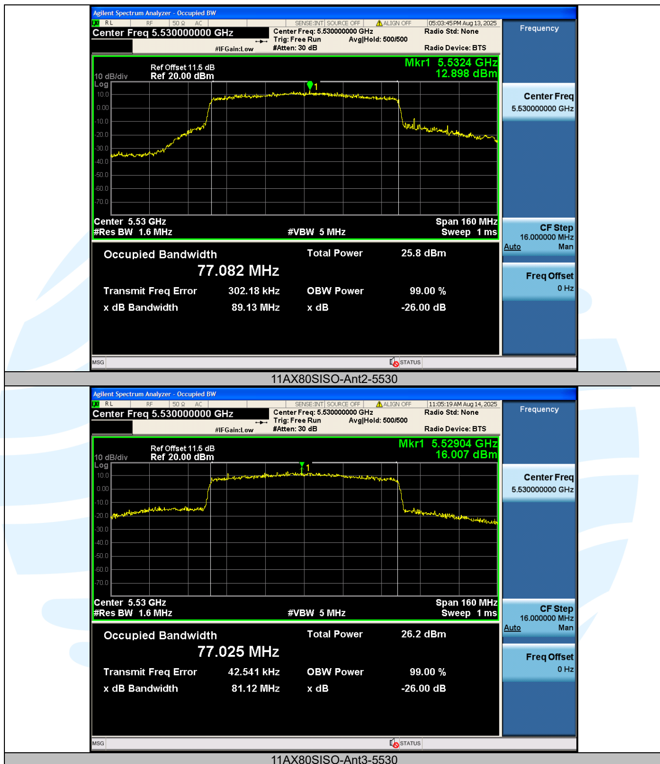
11AX80SISO-Ant3-5530
