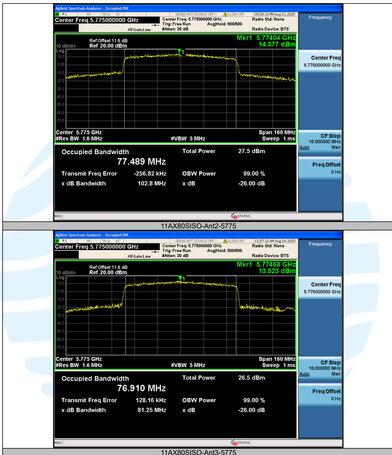
11AX80SISO-Ant3-5775
